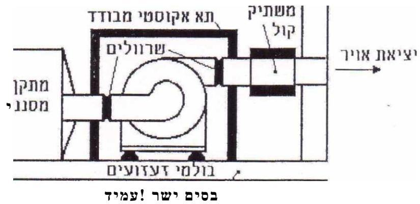
תרשים של אלמנטים למניעת רעש ורעידות ממפוח יניקה של מערכת סינון
