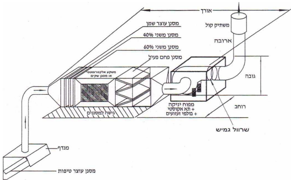
תרשים מס' 1 : מערכת אוורור וסינון לבתי אוכל
